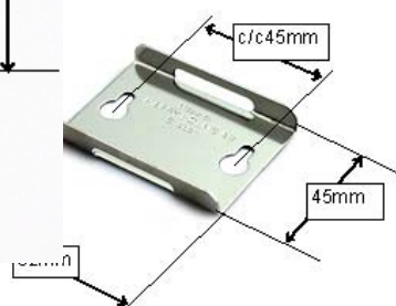
Kiinnitysosa pullotelineelle 8144
