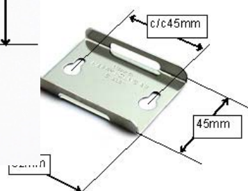
Kiinnitysosa pullotelineelle 8144
