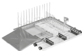
381 341 C Jäykkien skooppien pesuteline • sis. tiheän korin 381212 ja kannen 381213
